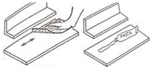
Sl. 6.21 - Čišćenje površina pre početka lemjenja
