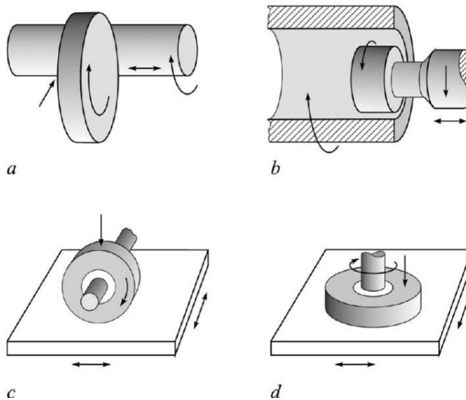
Поступак брушења
